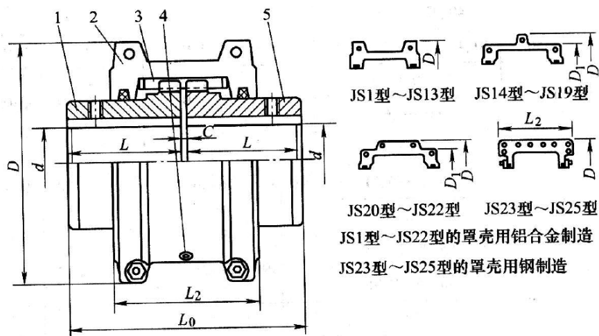
1、5—半联轴器 2—罩壳 3—蛇形弹簧 4—润滑孔
